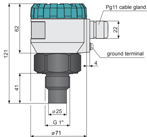
ULM-70_-02-I
