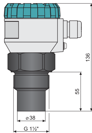
ULM-70_-06-I
