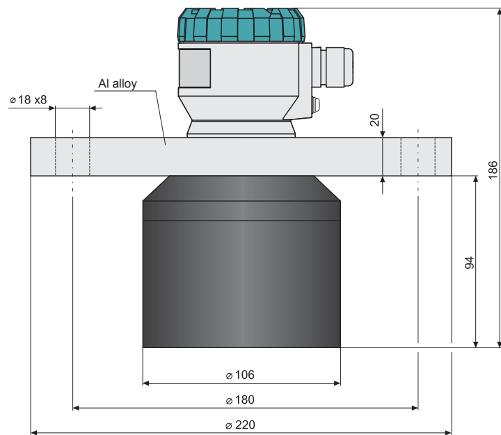
ULM-70_-20-I
