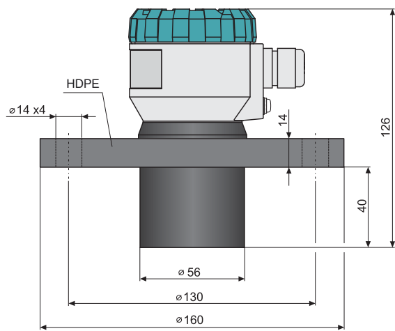
ULM-70N-10-I
