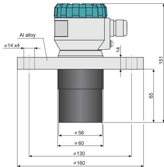
ULM-70Xi-10-I
